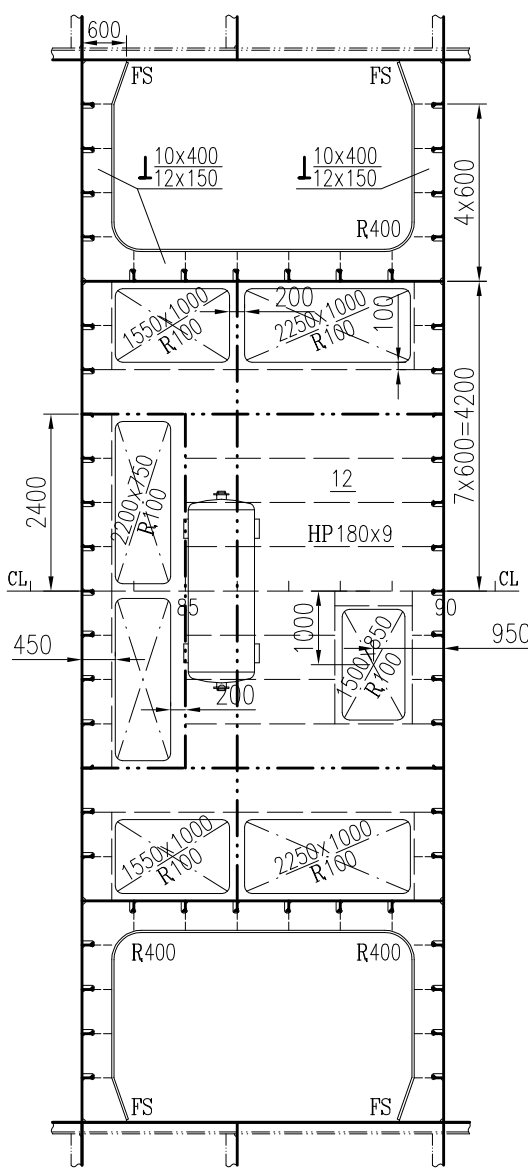
8070 STINGER 1:100
